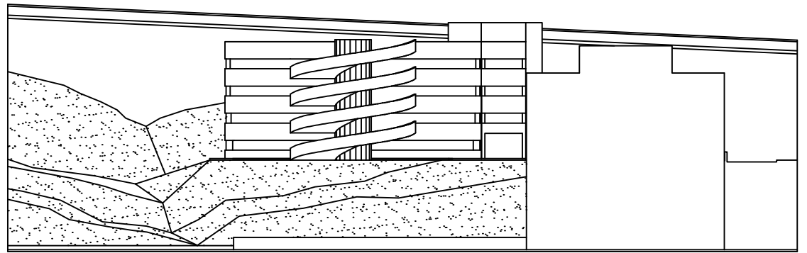
PROSPETTO SUD
