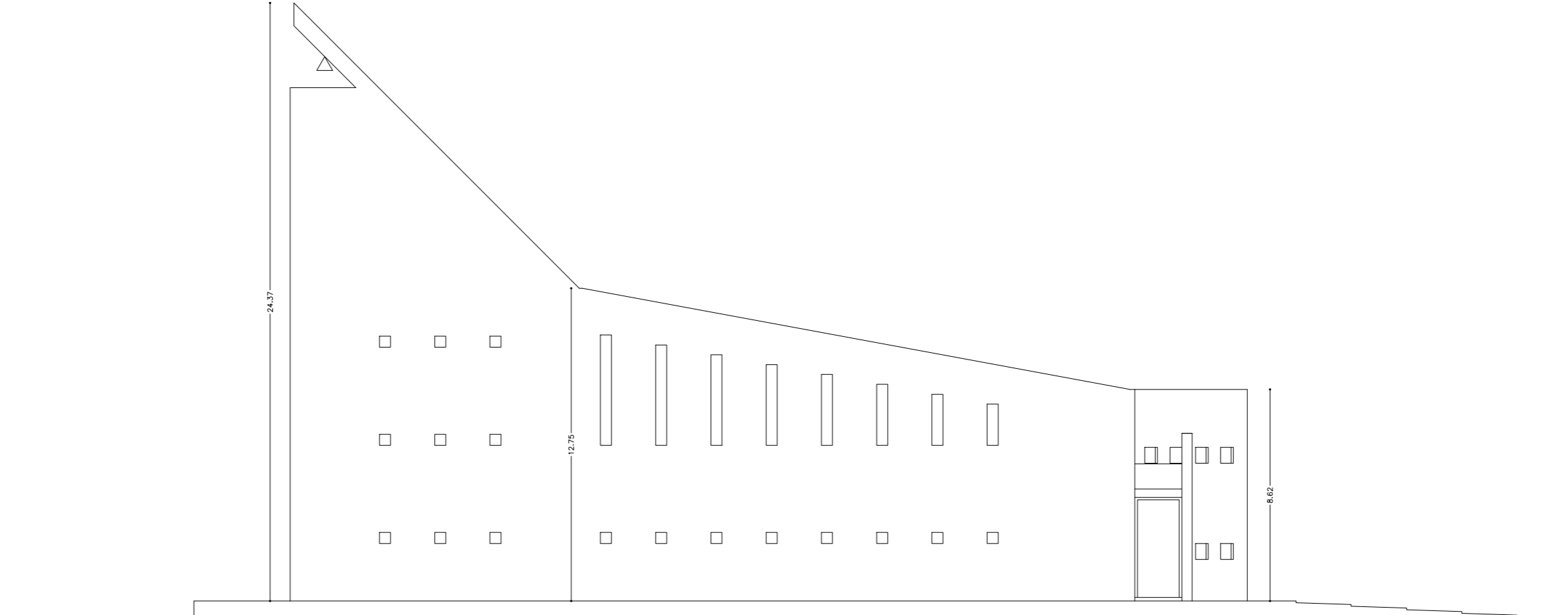
PROSPETTO EST
